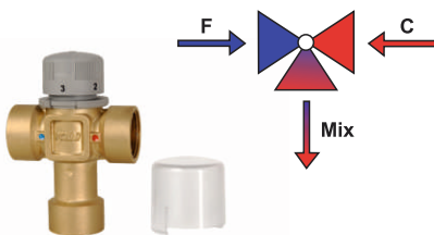
Trokraki mešni ventil "Icma" art. 149 Dimenzije: 1/2"; 3/4"; 1" Max pritisak: 10 bar Max temperatura: 85°C Temp. podešavanje: 30-65°C Pakovanje na kom.
