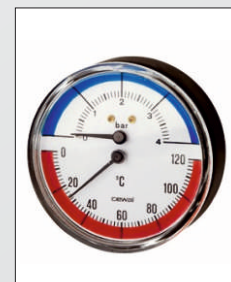
Termomanometar ABS Temperatura 0 - 120°C Pritisak 4 bar Axialni priključak Dimenzija: Ø 80 - 1/2"
