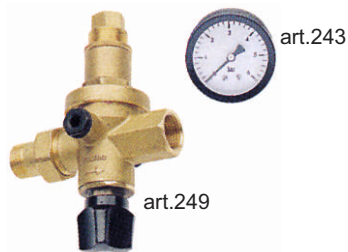
Automatski dopunjač sistema sa i bez manometra (6 - 16 bara) "Icma" Artikal 249 + 243 i artikal 249 Dimenzija: 1/2" Pakovanje na kom.
