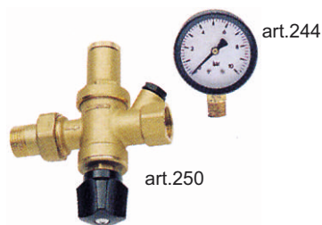
Automatski dopunjač sistema sa i bez manometra (3 - 10 bara) "Icma" Artikal 250+244 i artikal 250 Dimenzija: 1/2" Pakovanje na kom.
