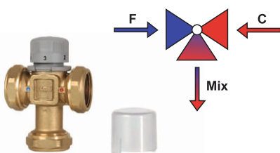
Trokraki mešni ventil "Icma" art. 163 Dimenzije: 22mm Max pritisak: 10 bar Max temperatura: 85°C Temp. podešavanje: 30-65°C Pakovanje na kom.
