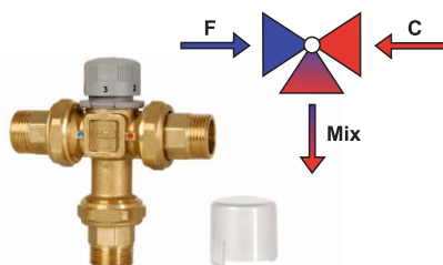
Trokraki mešni ventil "Icma" art. 148 Dimenzije: 1/2"; 3/4"; 1" Max pritisak: 10 bar Max temperatura: 85°C Temp. podešavanje: 30-65°C Pakovanje na kom.
