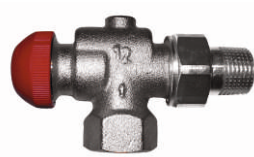
Usponski gornji ventil sa termostatskom opcijom i usponski gornji ventil TS set "Herz" (ventil sa termostatskom opcijom + termo glava STANDARD) Dimenzija: 1/2" Pakovanje: 10/20kom.
