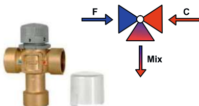
Trokraki mešni ventil "Icma" art. 149
