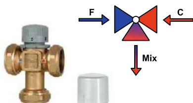
Trokraki mešni ventil "Icma" art. 163
