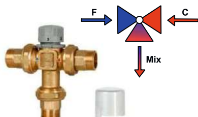
Trokraki mešni ventil "Icma" art. 148
